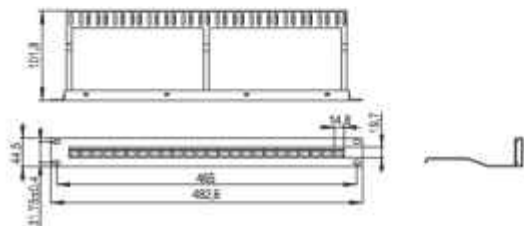
Рисунок/Figure 1 – PP24-11UMU
