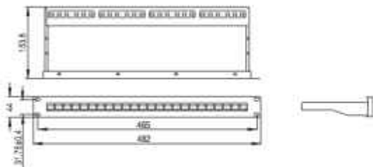
Рисунок/Figure 3 – PP2M-1UMF
