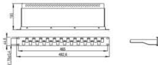
Рисунок/Figure 2 – PP24-11UMU-D
