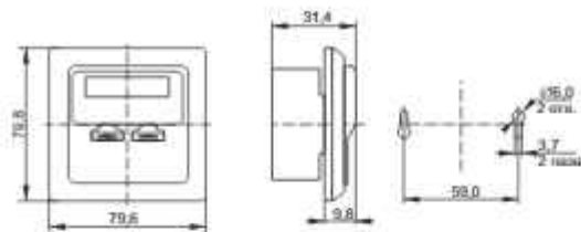
Рисунок / Figure 1 – Розетки / Jacks CS2-1CSEU-2-1, CS2-1C06U-2-1
