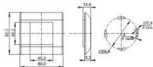
Рисунок / Figure 6 – Рамка / Frame CSS-12M-M
