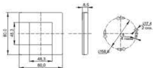
Рисунок / Figure 7 – Рамка / Frame CSS-12M-P
