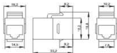
Рисунок / Figure 4 - Адаптер / Adapter CS7-1CSEF
