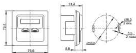
Рисунок / Figure 2 – Розетки / Jacks CS2-1C06F-2-1, CS2-1CSEF-2-1
