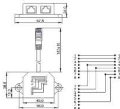
Рисунок / Figure 3 - Разветвитель / Splitter CS7-1CSEF, CS7-1CSEU
